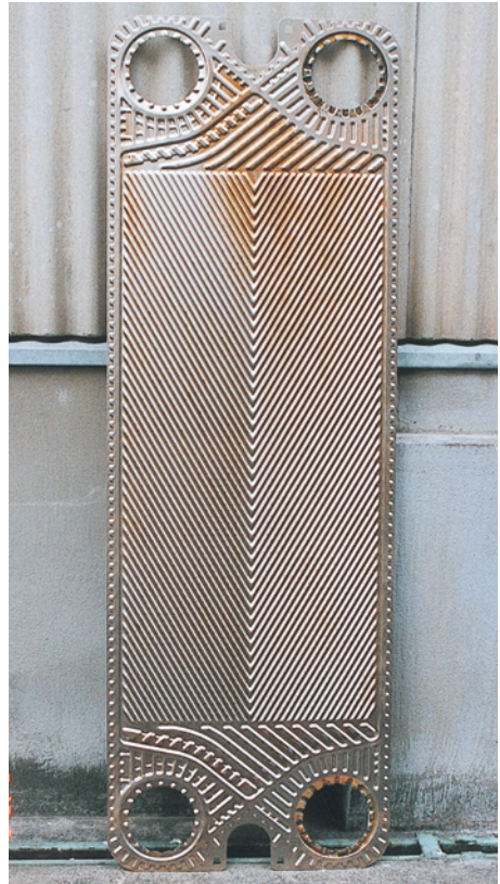
↑ Vapor side
